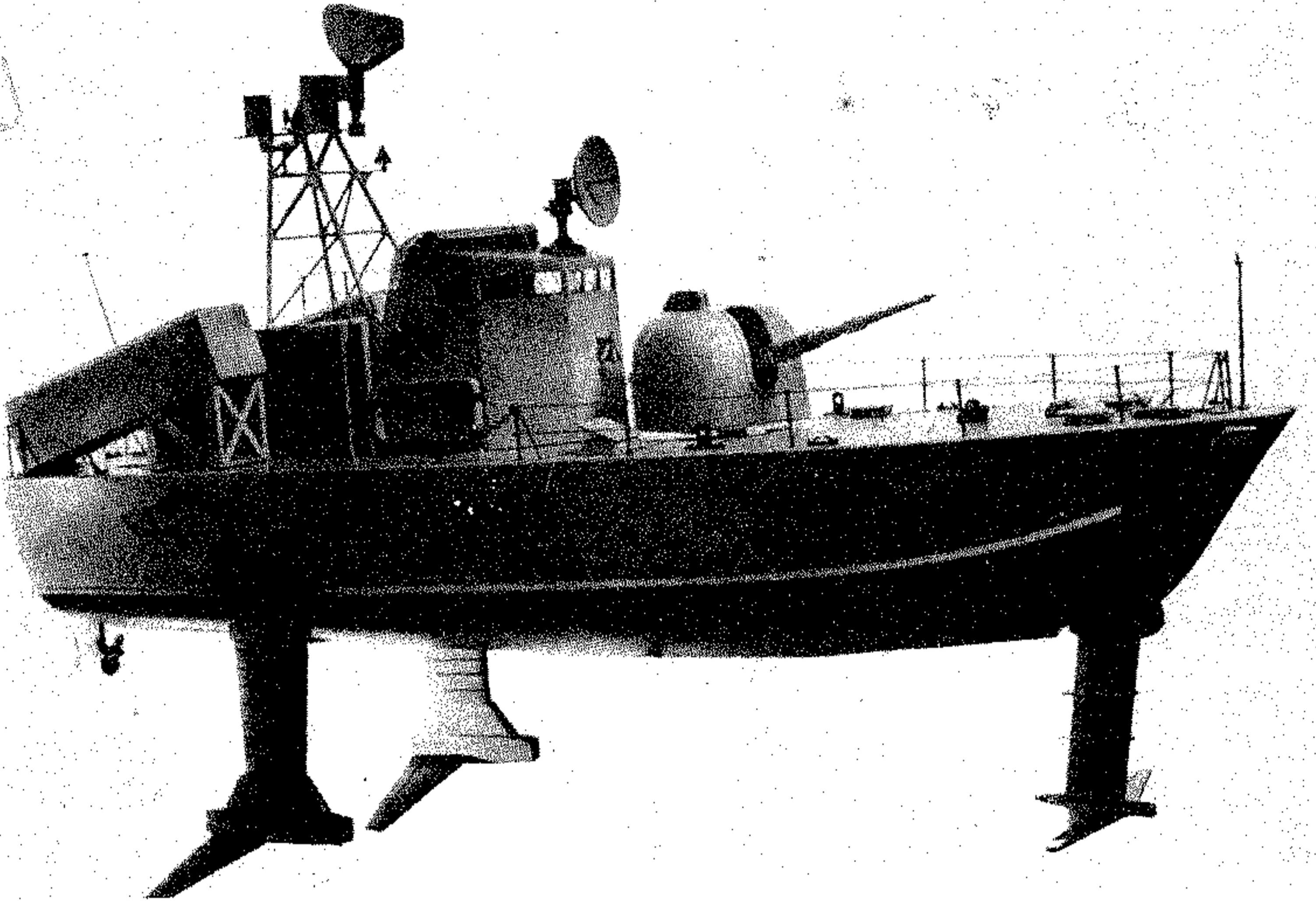
نموذج لزورق زلاقي إيطالي من فئة « سبارفييرو » . وهو يظهر الزلاقات التي تكون عادة غاطسة في الماء عند الابحار بسرعة كبيرة
