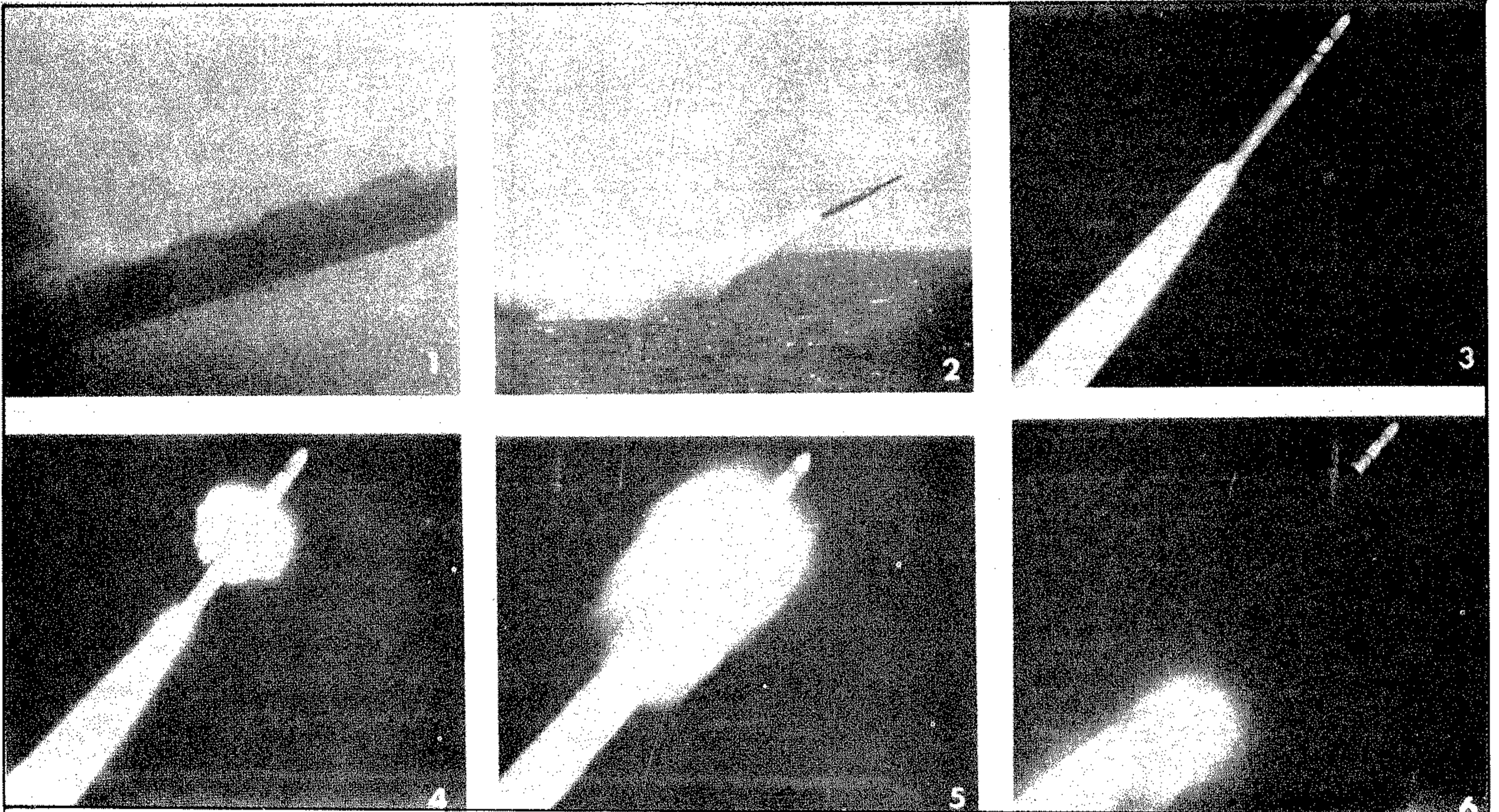
المراحل المتتابعة لمسار الصاروخ «سبروك»: ١ - الاطلاق من انبوب طوربيد الغواصة الموجودة تحت الماء. ٢ - خظة خروج الصاروخ من الماء إثر اشتعال محركه. ٣ - تسارع الصاروخ في الجو إلى ما فوق سرعة الصوت. ٤ و ٥ - قنبلة الأعماق النووية تنفصل عن المحرك الصاروخي. ٦ - لحظة توجه قنبلة الأعماق نحو الهدف بفعل نظام التوجيه
