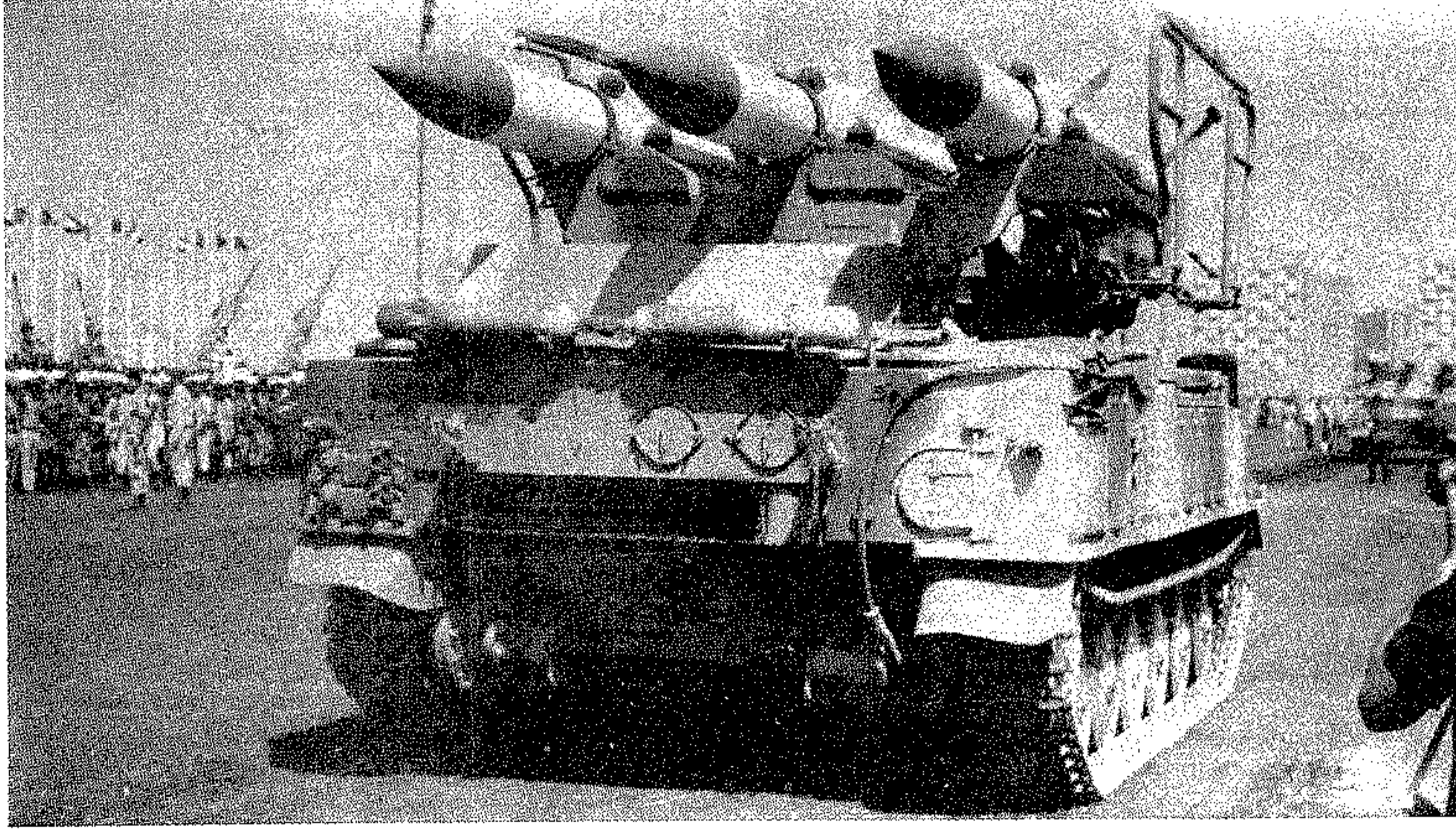
صواريخ سوفيتي رص - جو «سام - 6» عاينفول
