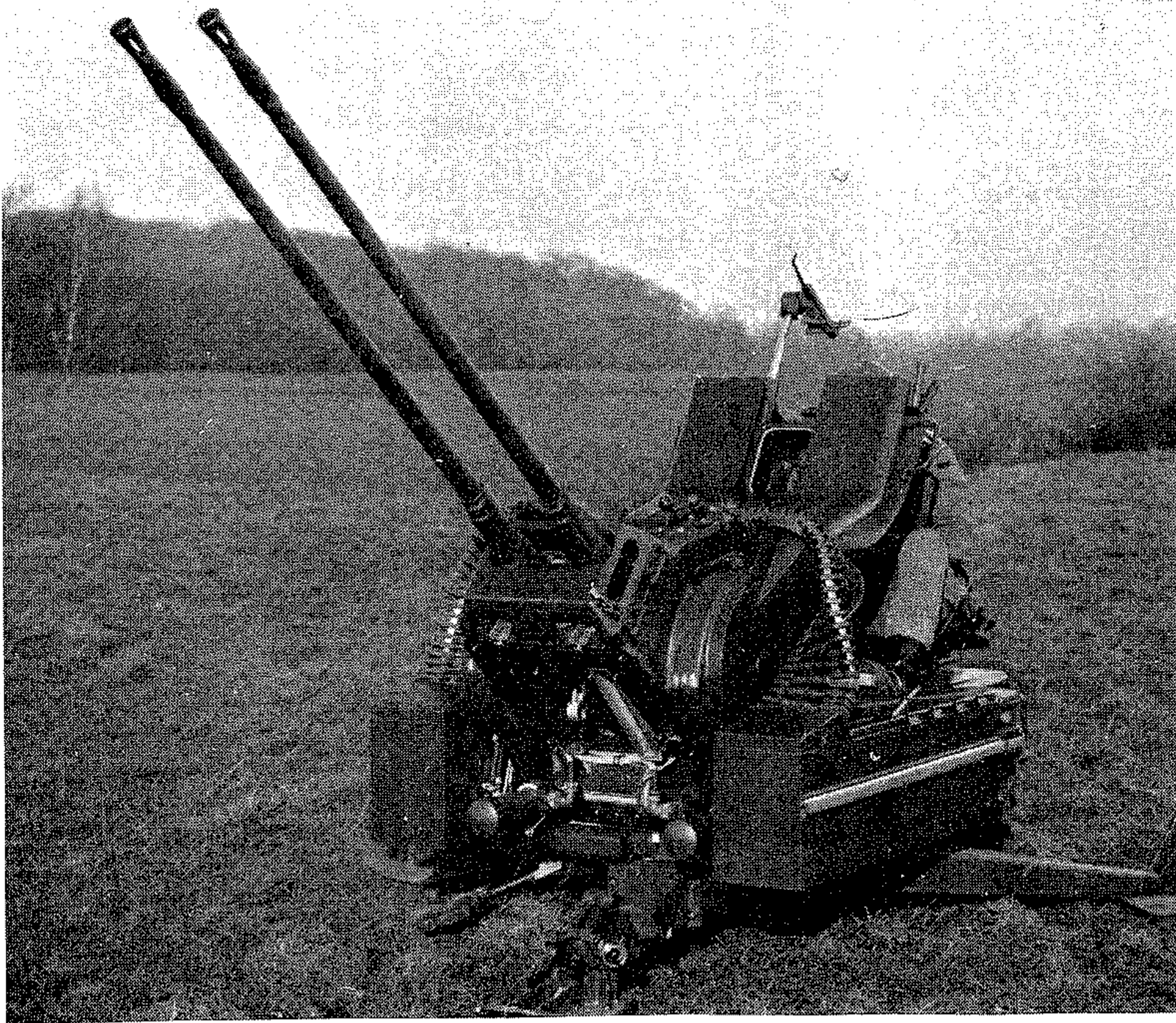
مدفع الماني غربي مضاد للطائرات من طراز « ر ه - ٢٠٢ » ثنائي السبطانات
