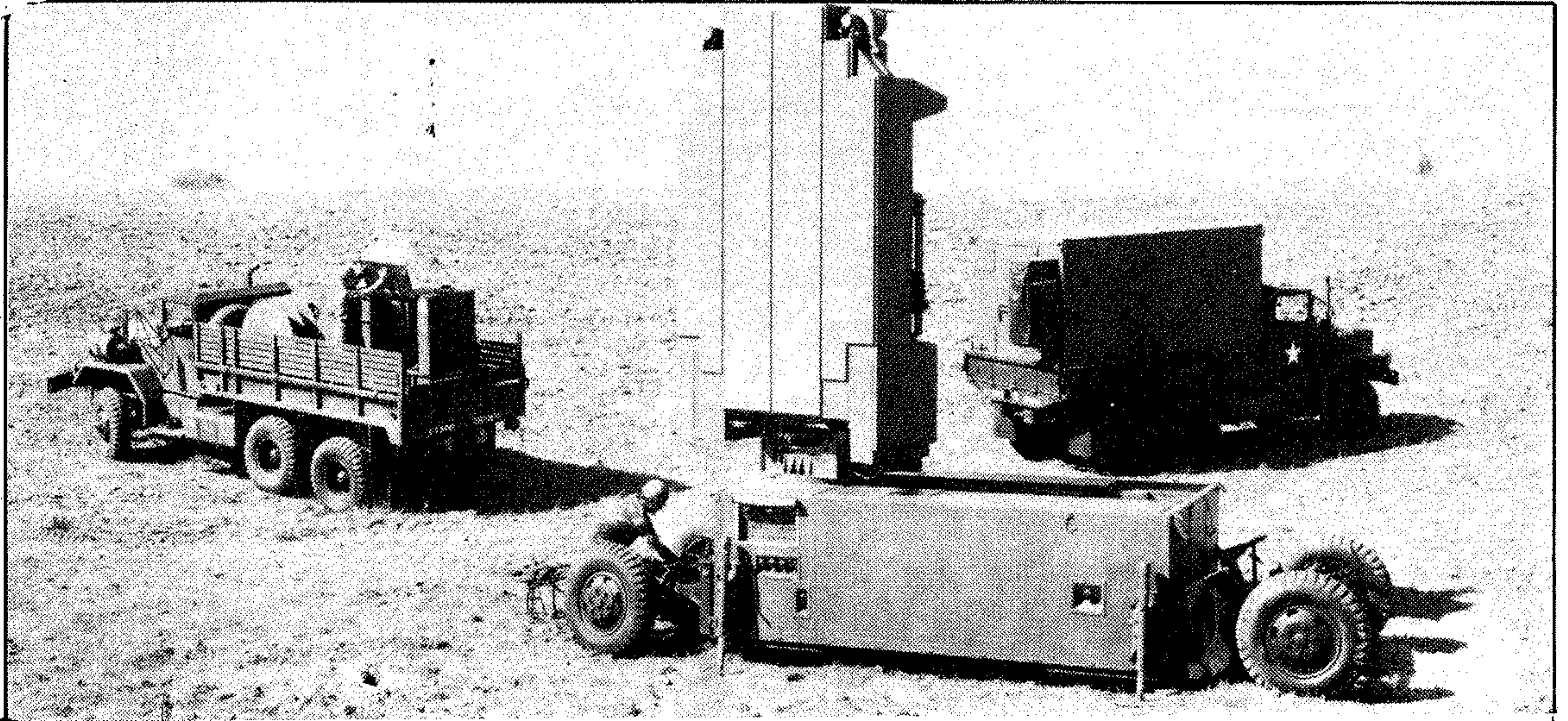
يتألف نظام الرادار «أن/ت ب كيو- ٣٧» من مقطورة تحمل الهوائي (في الوسط) ووحدة توليد الطاقة الكهربائية (إلى اليسار)، ومركز التشغيل والعمليات الذي تم منه ادارة الجهاز في الميدان (إلى اليمين).
