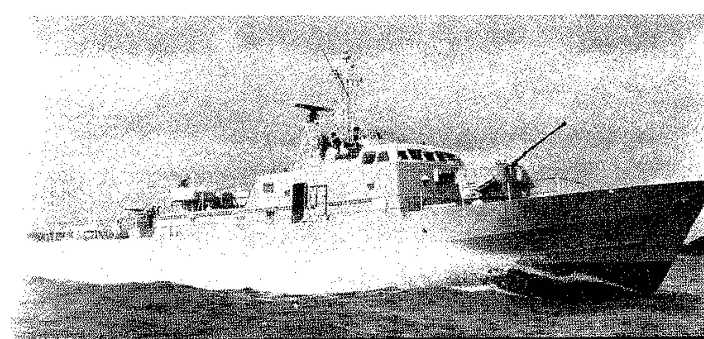
زورق هجوم سريع بريطاني مسلح بمدافع « ثوسپر ثورنيكروفت » طراز ( أ )
