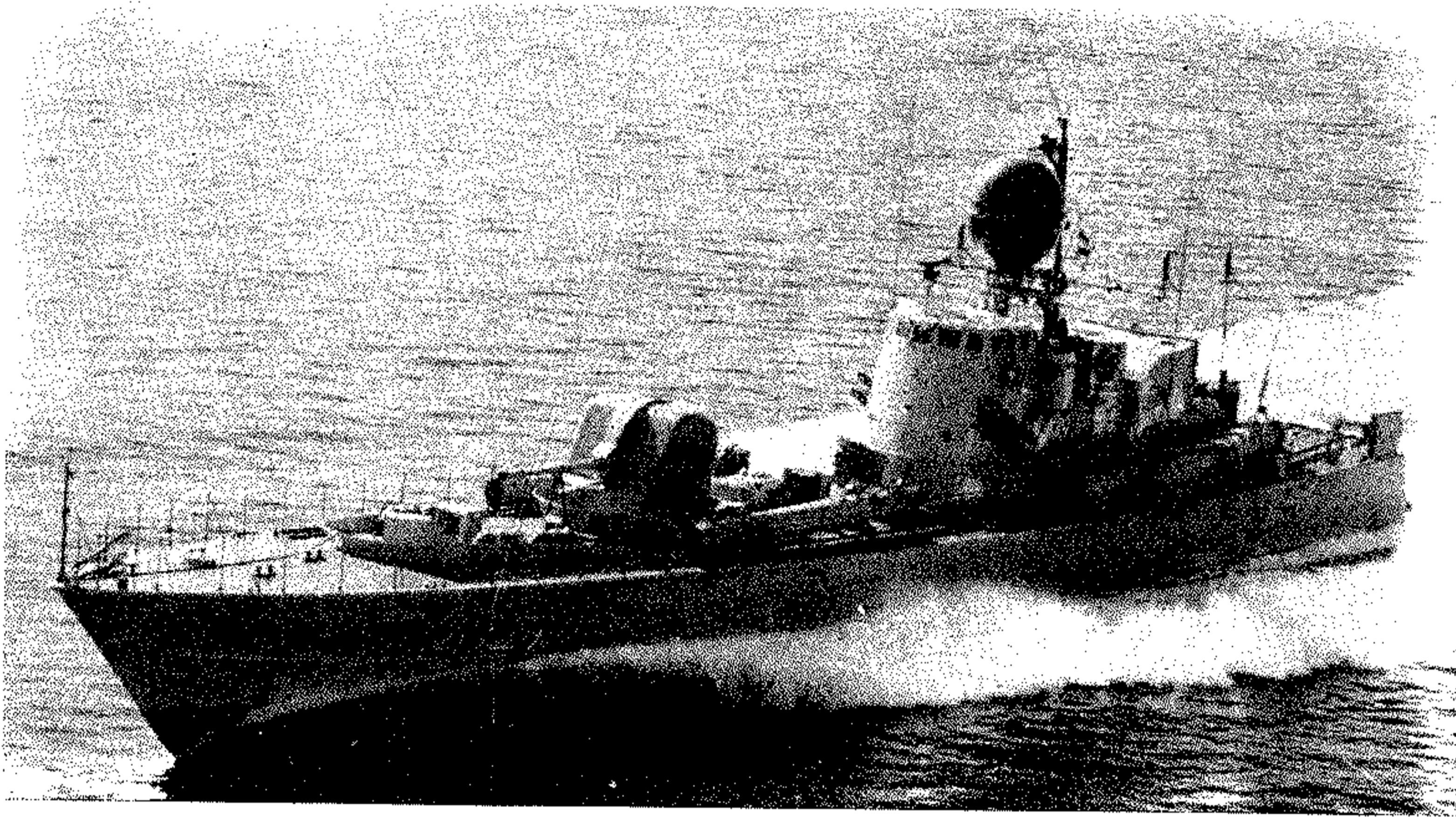
زورق هجوم سريع سويدي من طراز «سبيكا ت-١٢١»
