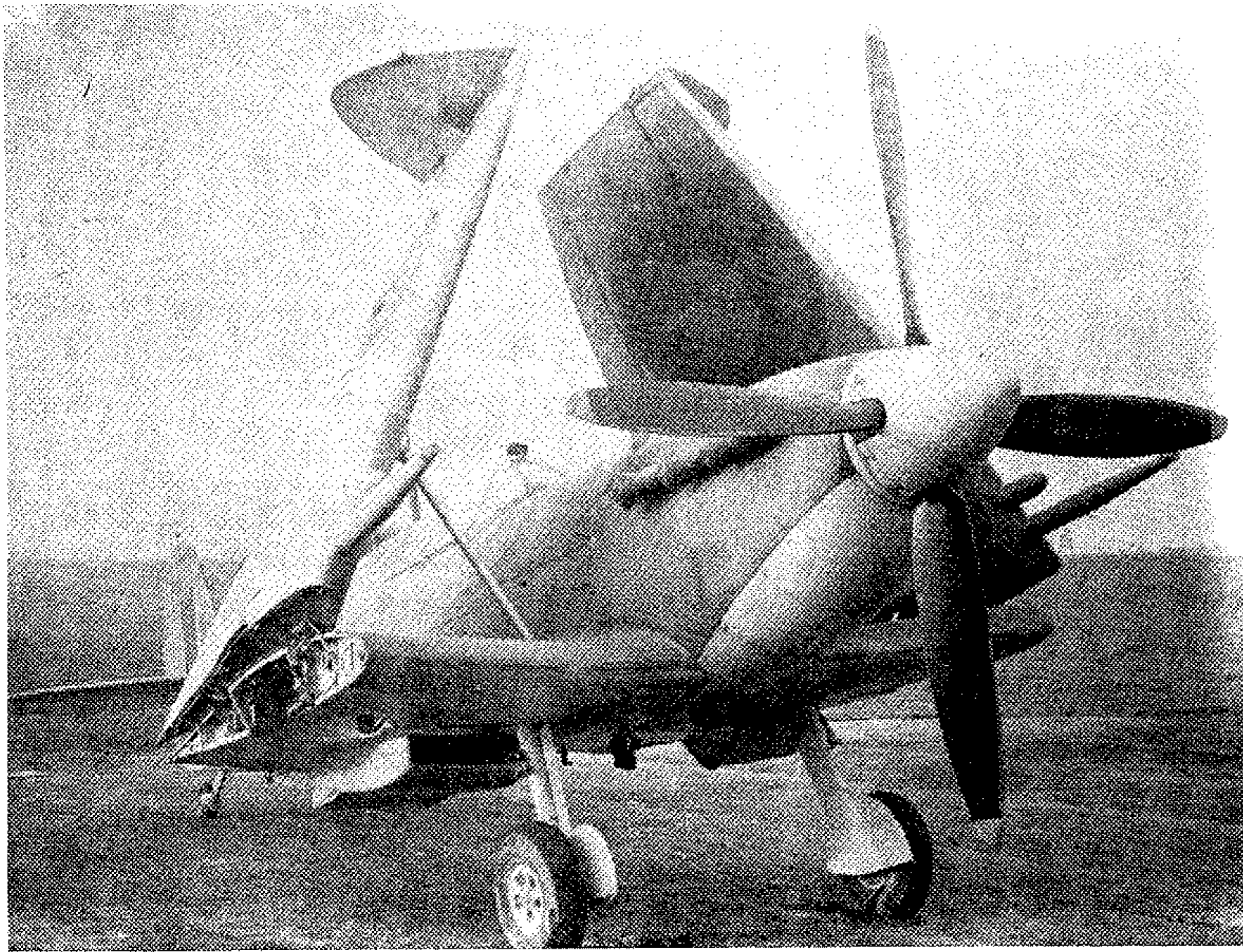
طائرة «سي فاير- ٣» ذات أجنحة قابلة للطي
