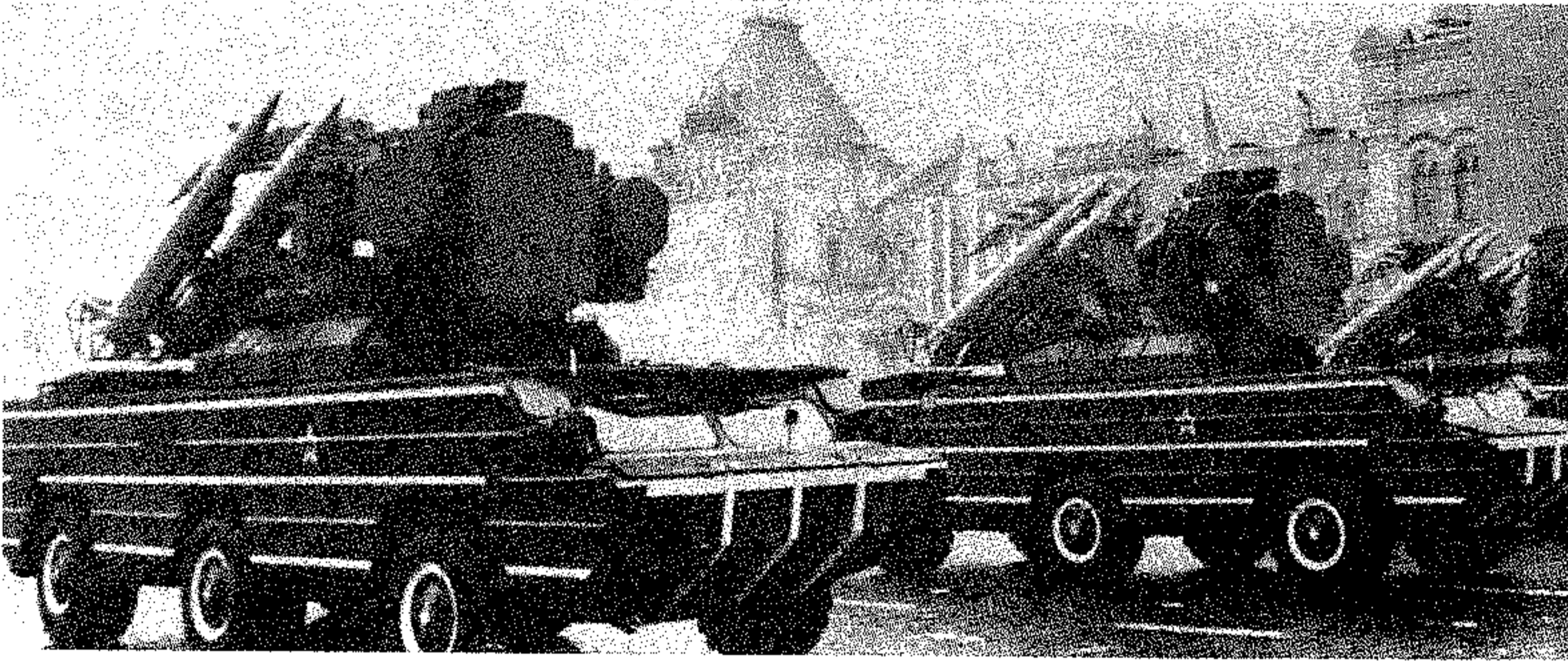
الصاروخ السوفياتي أرض - جو «سام - ٨ غيكو»
