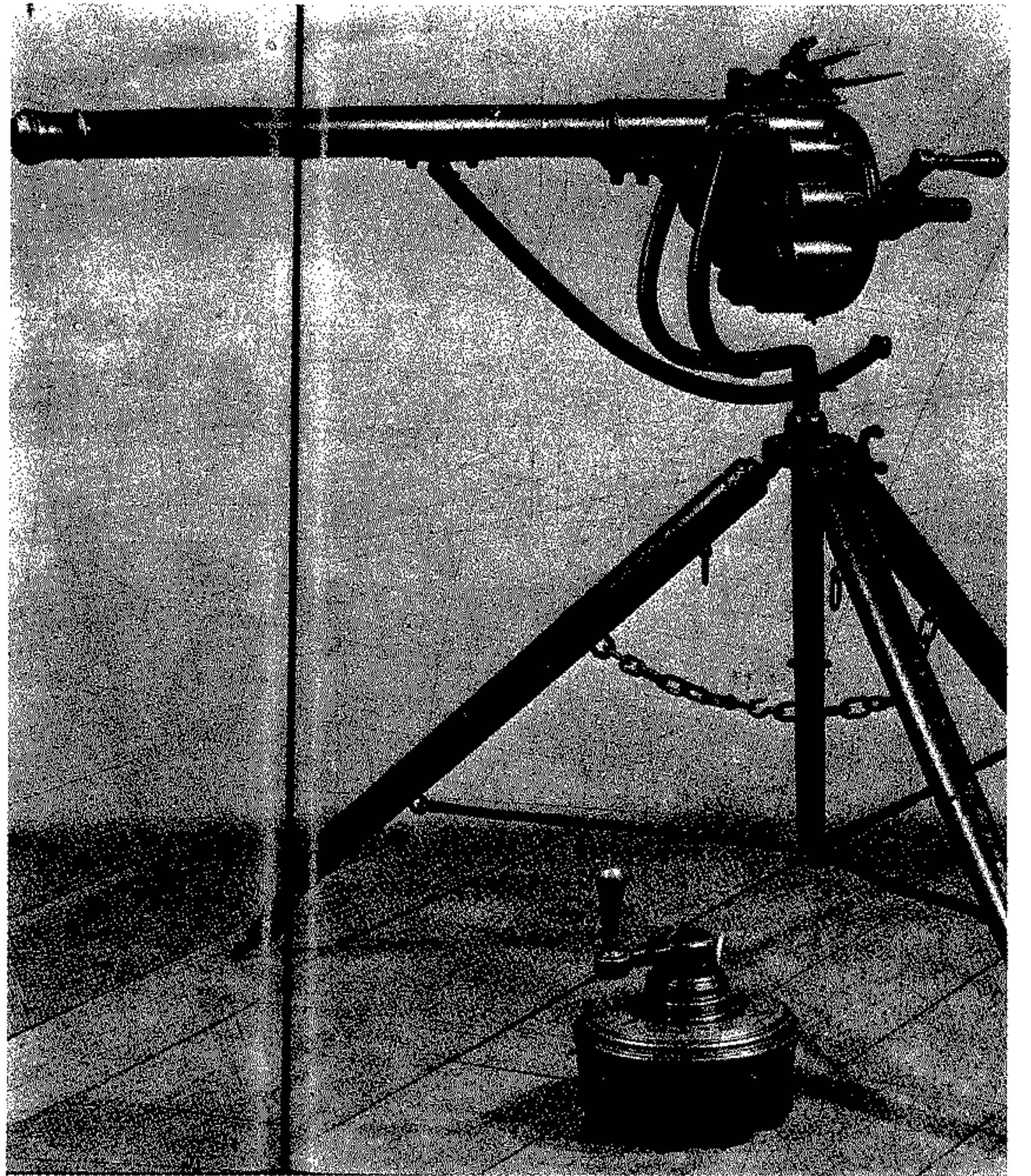
الرشاش الانكليزي « باكل »
