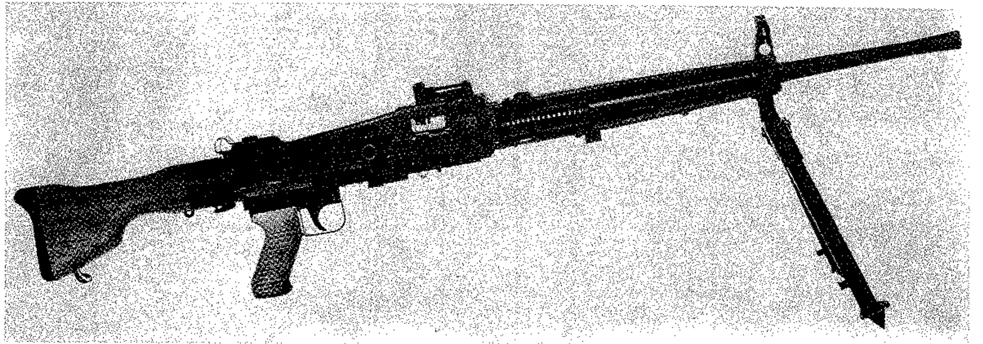
الرساس الخفيف السويسري « زيغ - ٧١٠ »
