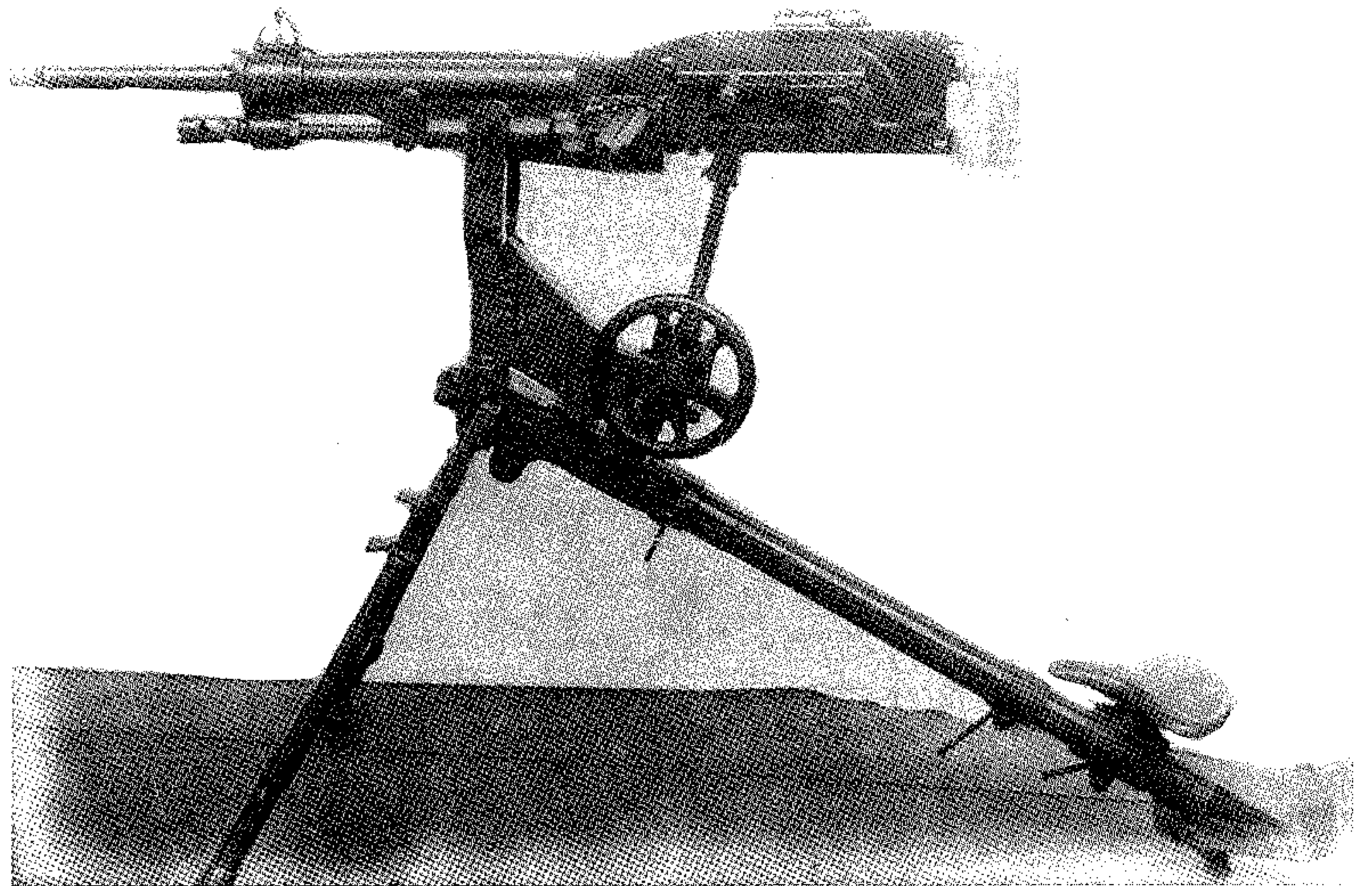
الرشاش الفرنسي سات إيتيين من عيار ٨ ملم (١٩٠٧)
