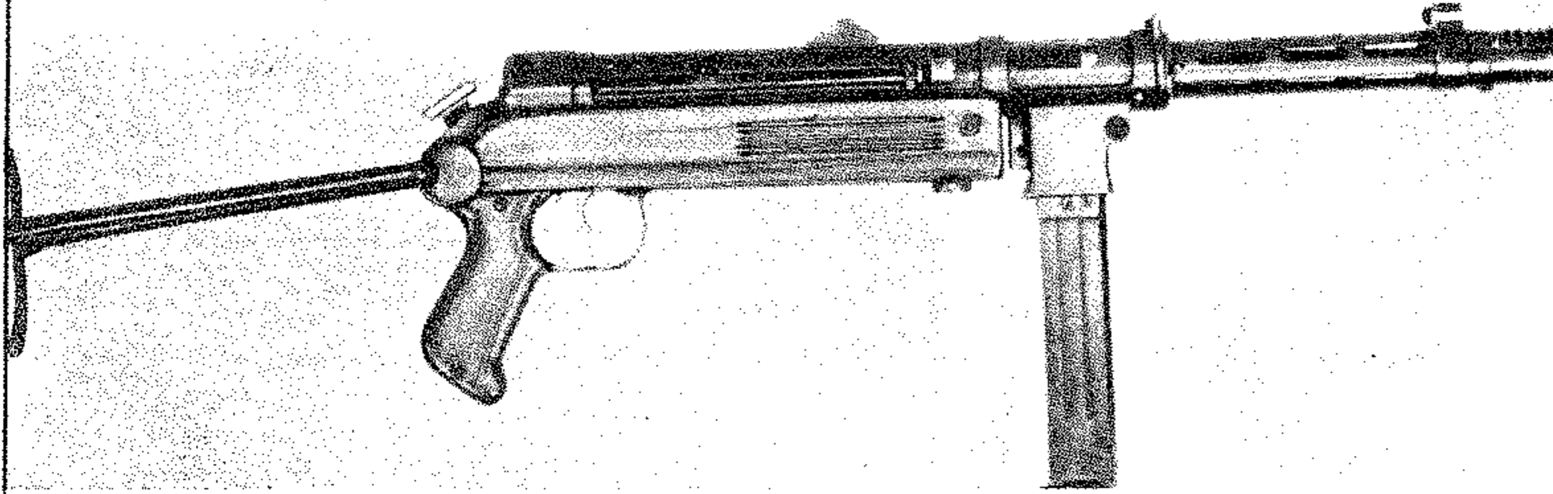
رشيثة « ستار » اسبانية من طراز « ز - ٤٥ »
