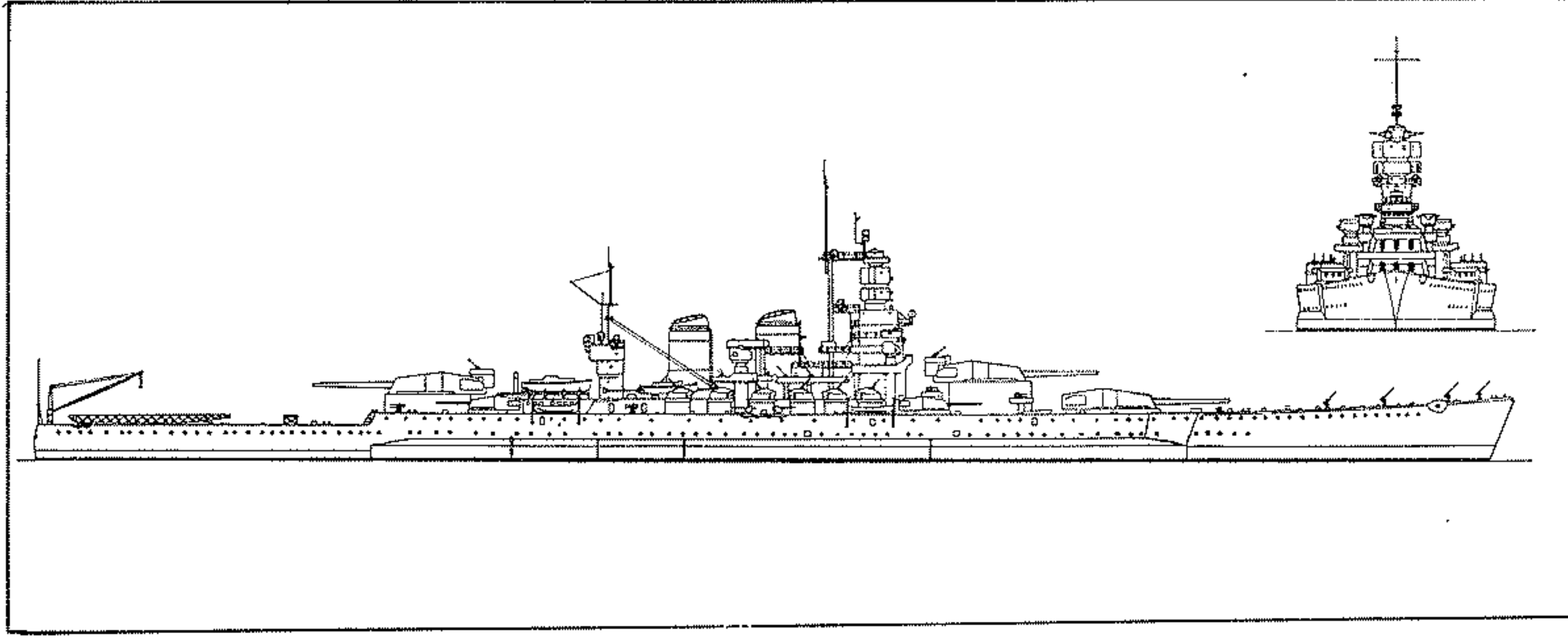
البارجة الايطالية « روما » من فئة « فيتوريو إيمانويل »
